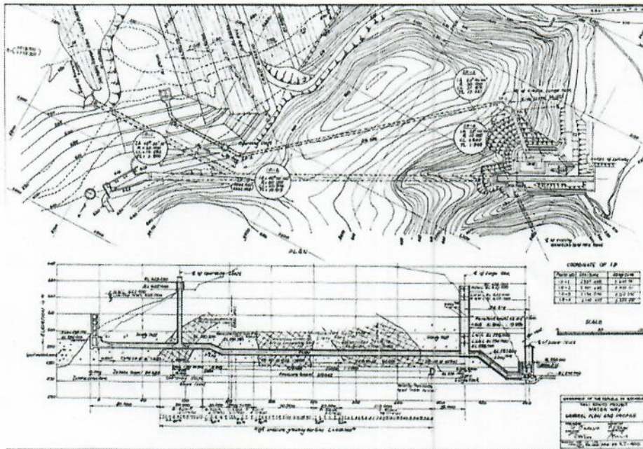
Gambar 3.1 Potongan Memanjang Waterway PLTA Selorejo
