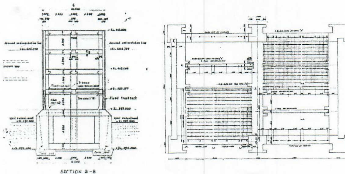
Gambar 3.1 Potongan Memanjang Waterway PLTA Selorejo
